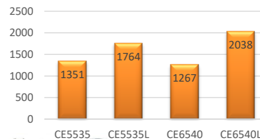
強度試験データ(kgf)1段積
